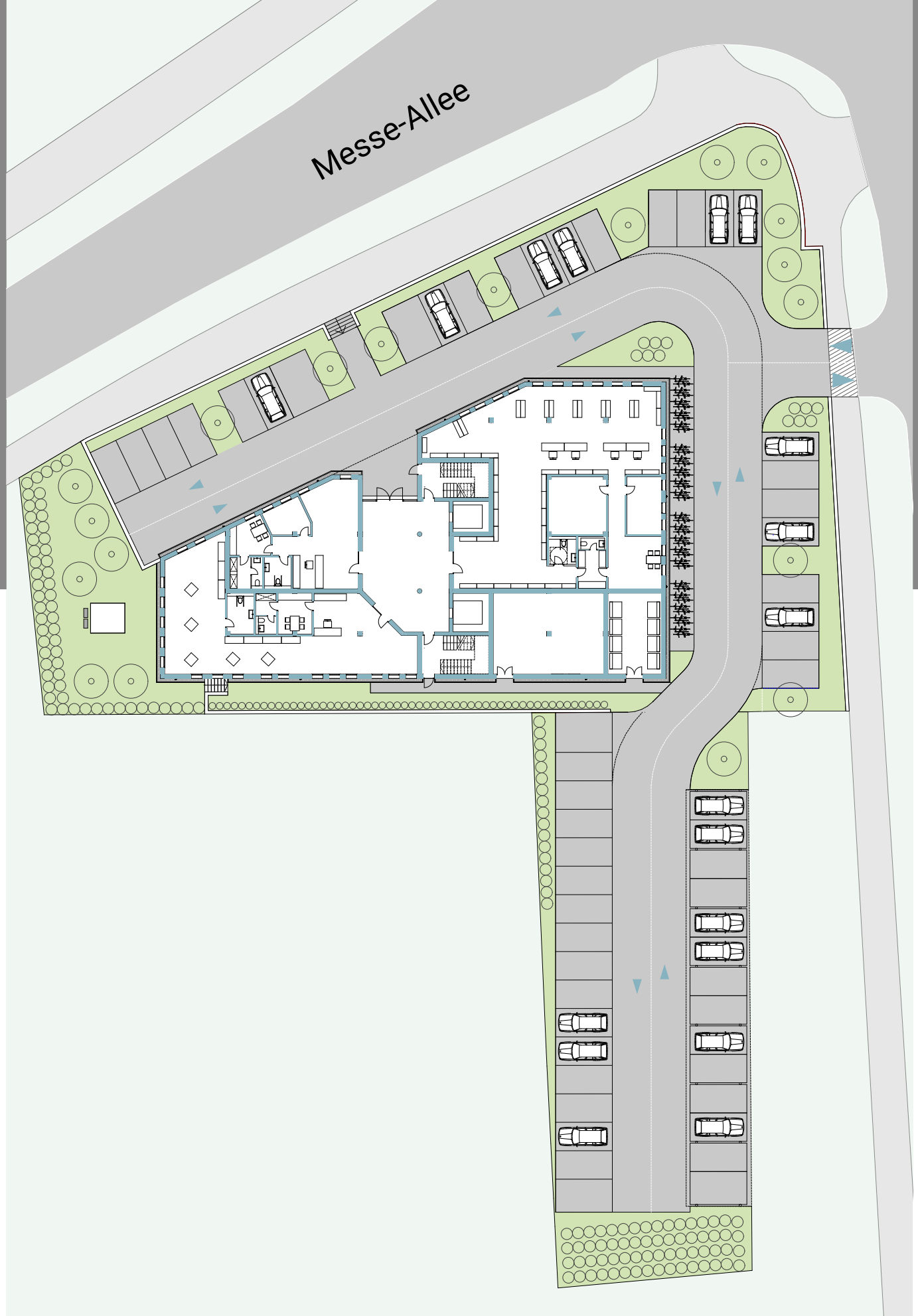
Freiflächenplan
